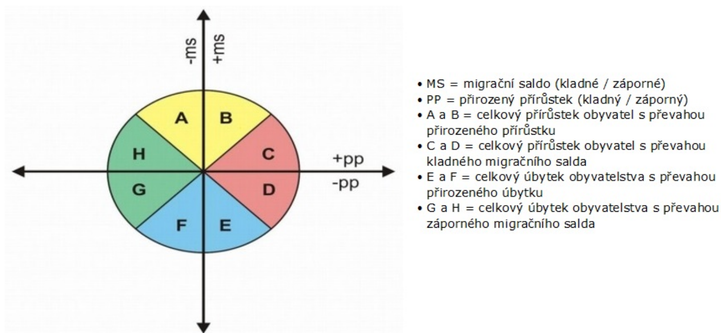
Obr. 2: Webbův diagram
