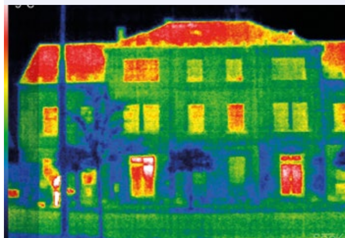
Termosnímek obecního úřadu obce Dolní Podluží slouží jako jeden ze zdrojů pro plánování energetické optimalizace
